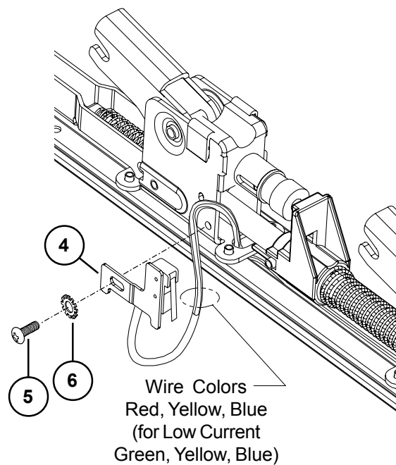
RX-AUX Switch
